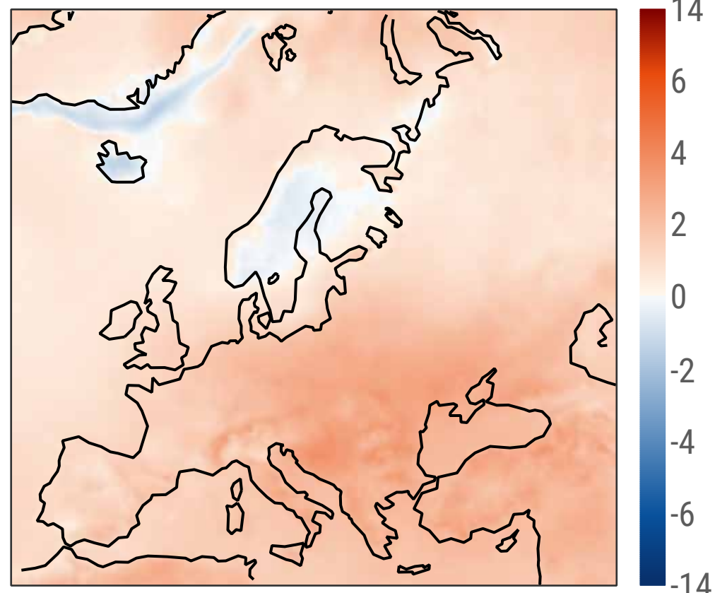
Surface air temperature (°C)
